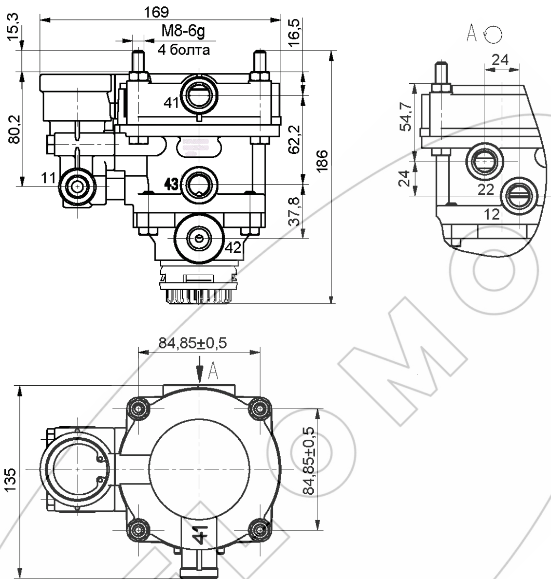
Рисунок 1 – Габаритные и присоединительные размеры клапана.
